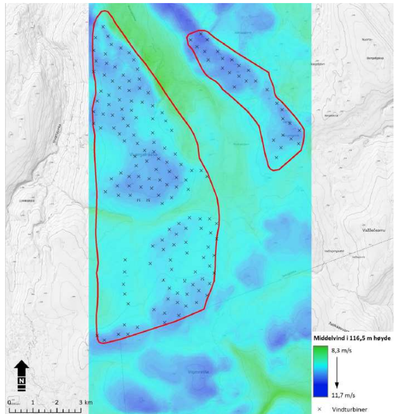
Govva 4: Lávvaguovllu bieggakárta. Gáldu: Kjeller Vindteknikk.
